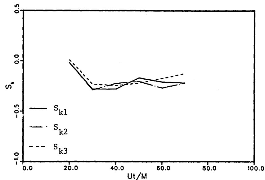
Velocity-Derivative Skewness
