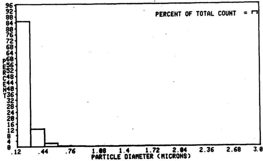
Fig. 18. Cigarette Smoke
