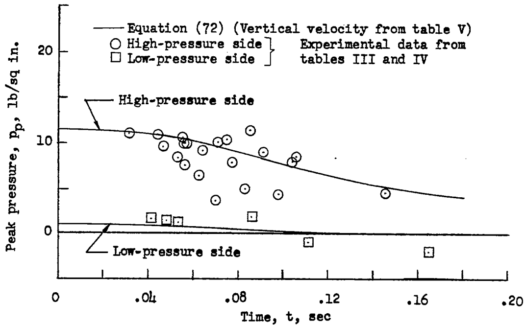
(a) Run 5: \tau = 3.2^\circ ; \psi = 12^\circ ; \dot{x}_0 = 71.5 feet per second; \dot{z}_0 = 4.2 feet per second.
