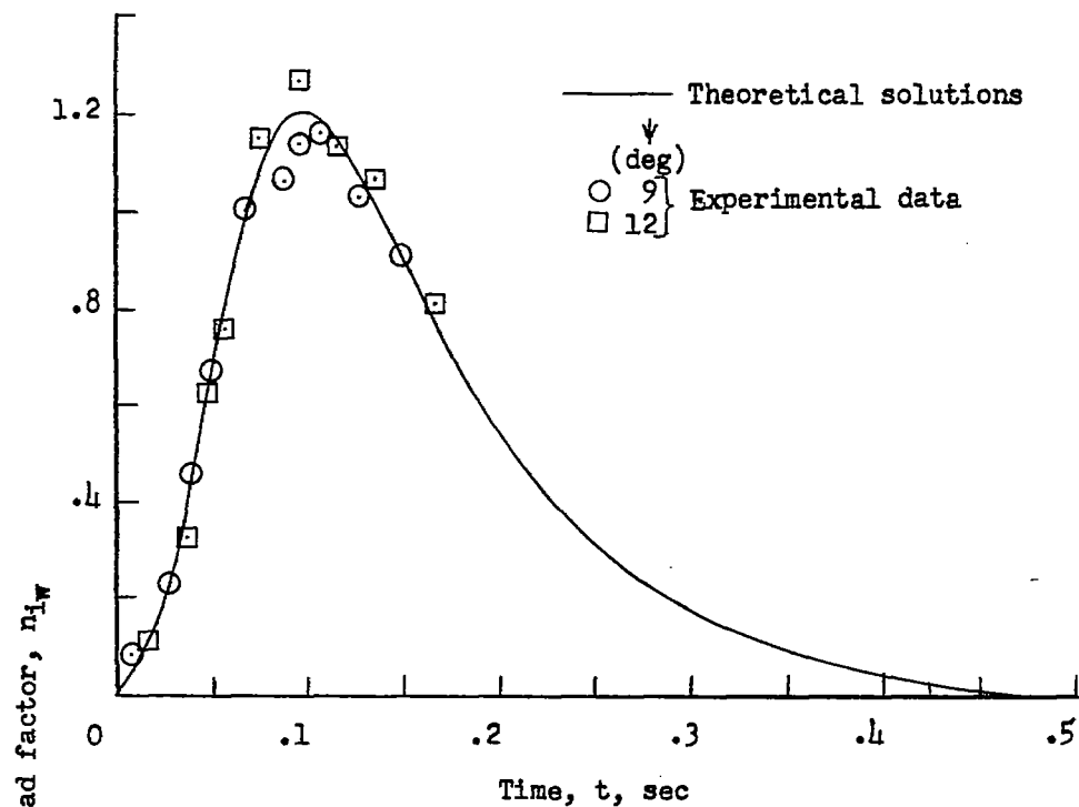
(a) \tau = 3.2^\circ ; \dot{z}_0 = 4.2 feet per second; \dot{x}_0 = 71.5 feet per second.
