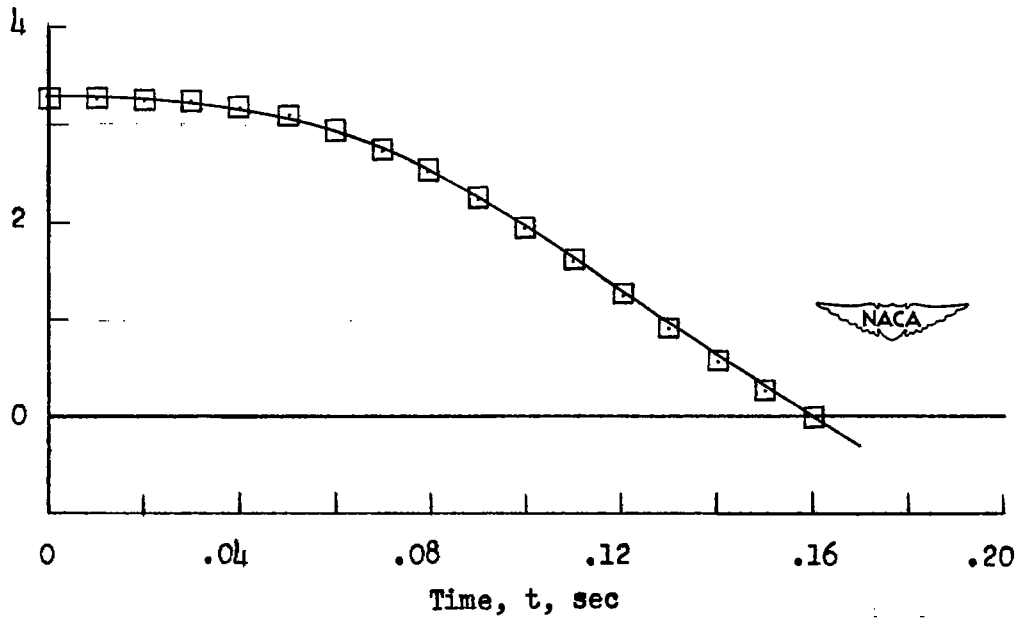
(b) \tau = 9.3^\circ ; \dot{z}_0 = 3.3 feet per second; \dot{x}_0 = 67.1 feet per second.
