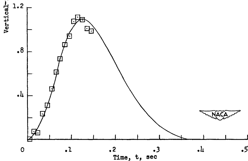
(b) \tau = 9.3^\circ ; \dot{z}_0 = 3.3 feet per second; \dot{x}_0 = 67.1 feet per second.
