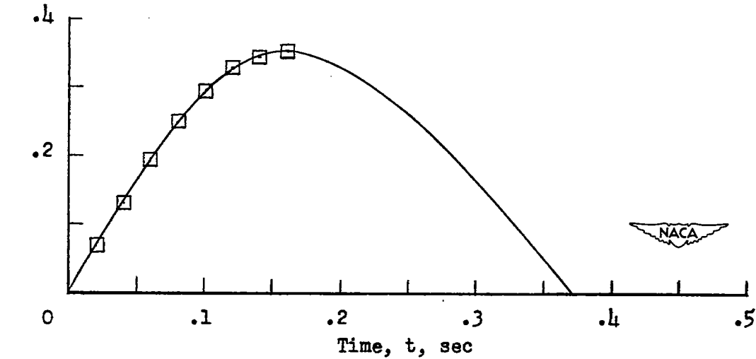
(b) \tau = 9.3^\circ ; \dot{z}_0 = 3.3 feet per second; \dot{x}_0 = 67.1 feet per second.
