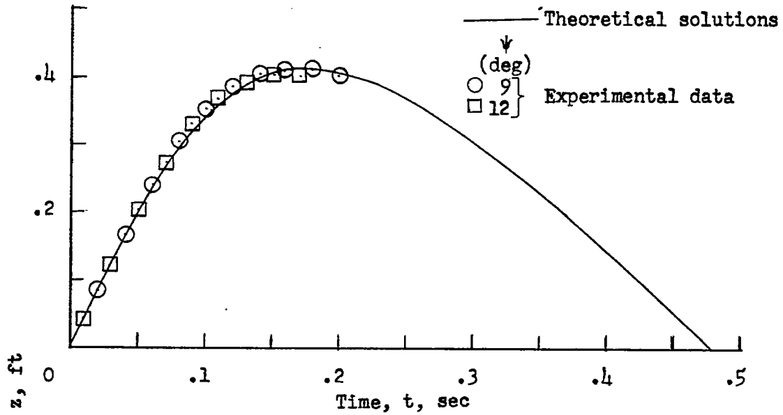
(a) \tau = 3.2^\circ ; \dot{z}_0 = 4.2 feet per second; \dot{x}_0 = 71.5 feet per second.
