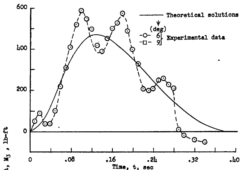
(a) \tau = 9.3^\circ ; \dot{z}_0 = 4.2 feet per second; \dot{x}_0 = 57.8 feet per second.
