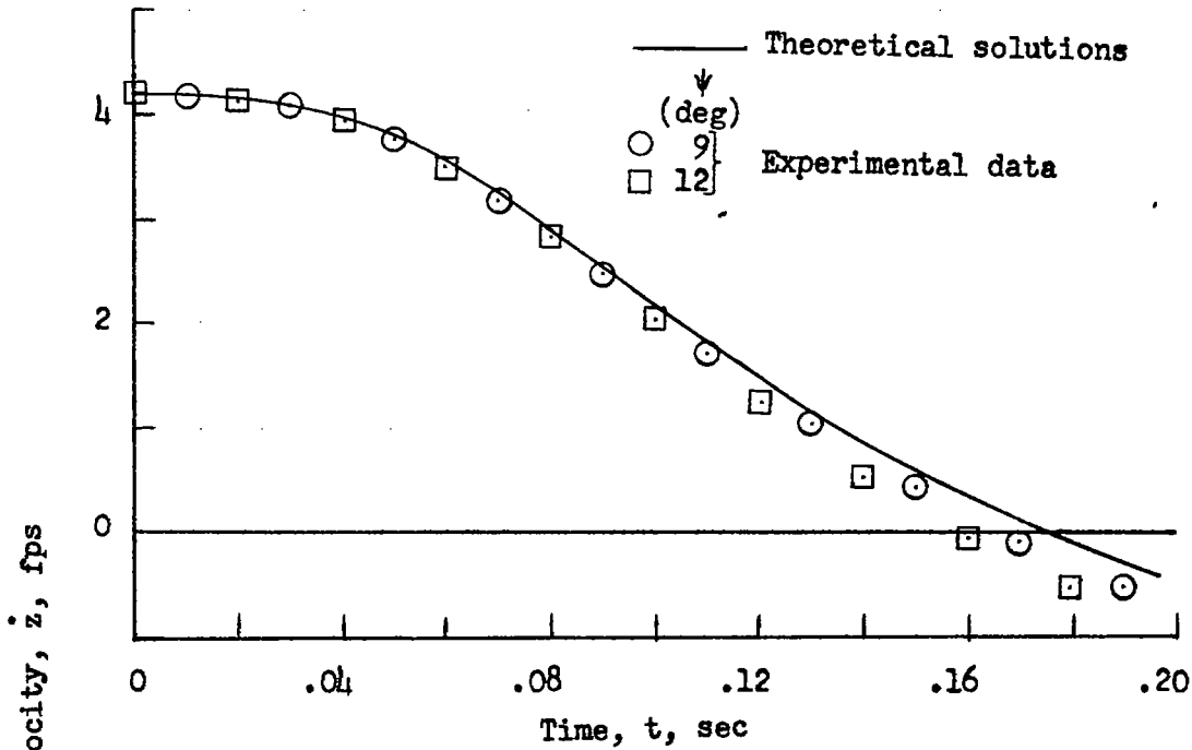
(a) \tau = 3.2^\circ ; \dot{z}_0 = 4.2 feet per second; \dot{x}_0 = 71.5 feet per second.
