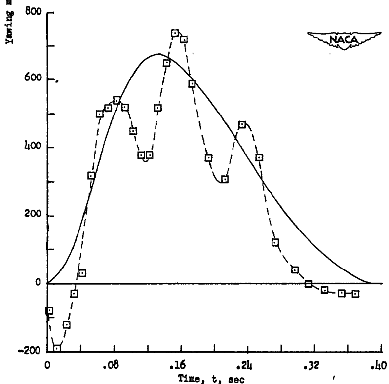
(b) \tau = 9.3^\circ ; \dot{z}_0 = 4.1 feet per second; \dot{x}_0 = 56.6 feet per second.
