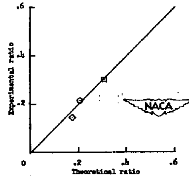
(d) Ratio of side to normal force, F_{\eta}/F_{\xi} .
