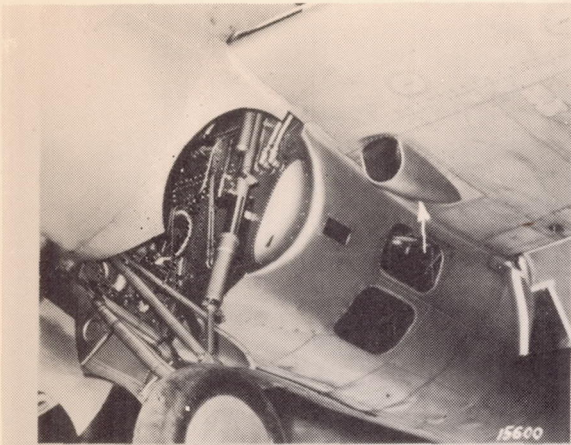
Inlet.
