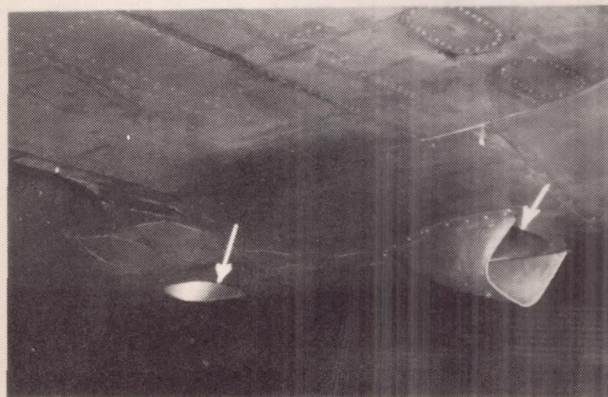
(d) Airplane 8.
