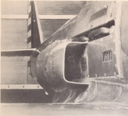
Inlet.
