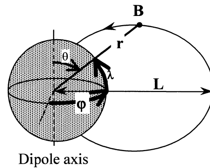
Fig. 25. Magnetic coordinates
