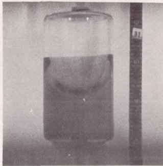
(b-1) Alcohol (contact angle, 0^\circ ).
