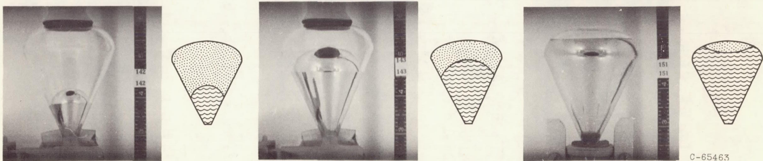
(c-3) Mercury (contact angle, 125^\circ ).
