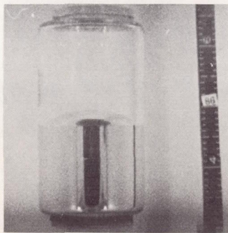
(b-3) Mercury (contact angle, 125^\circ ).
