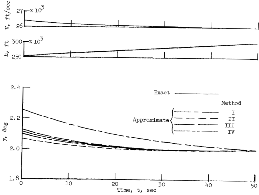
(d) V_d = 26,000 ft/sec; \gamma_d = 2^\circ ; C_L = -0.5 .
