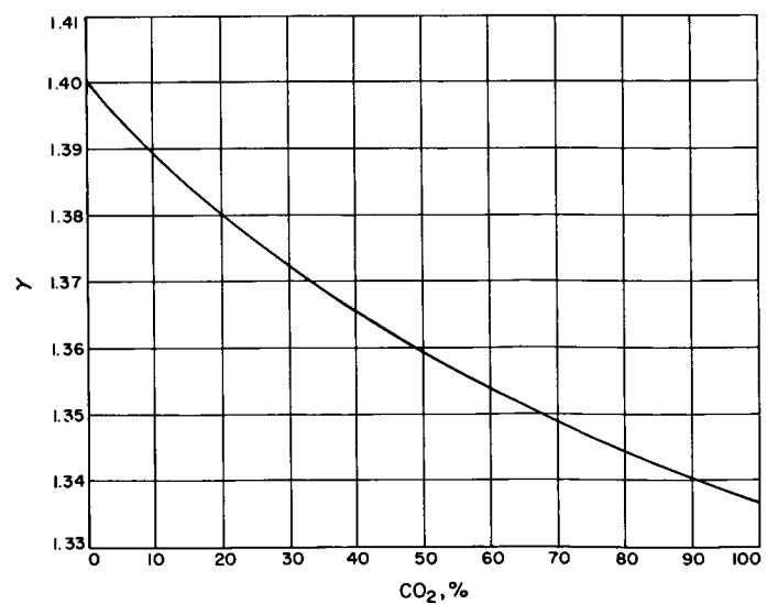
Fig. 9. \gamma vs % \text{CO}_2
