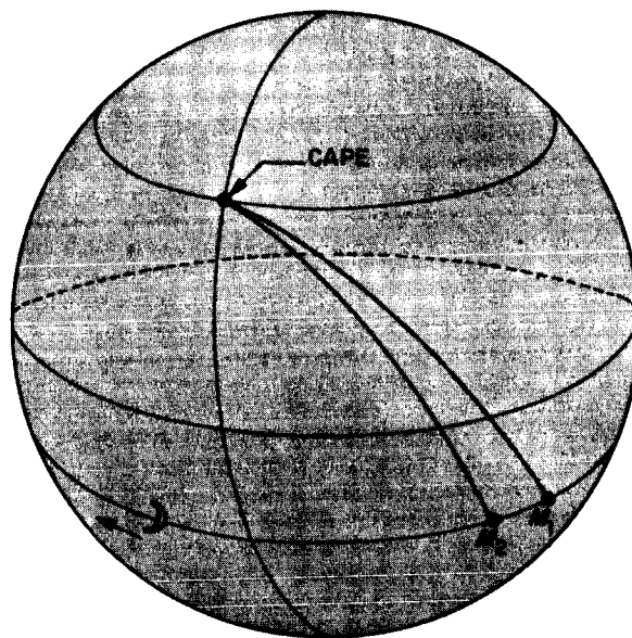
Fig. 5. Geocentric trajectories
