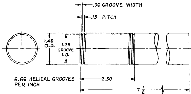
ITEM (16) -021 COIL FORM FOR ITEM (1), (2) & (3) -006 -007 & -008
