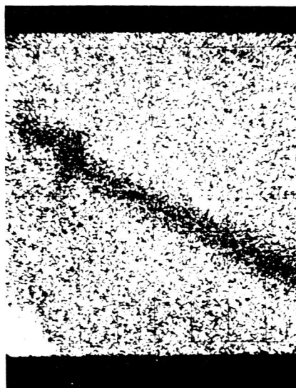
FeK \alpha
