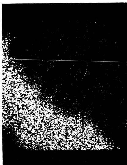
CrK \alpha
