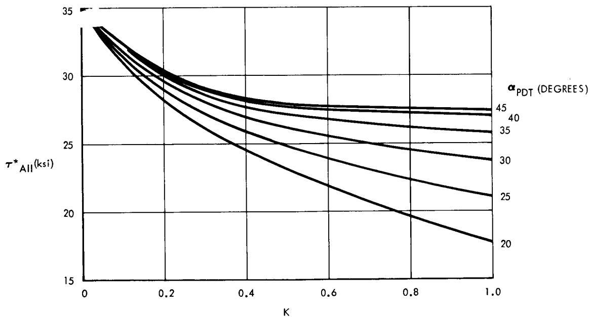
B ALCLAD 75S-T6 ALUMINUM ALLOY. \sigma_{tu} = 72 ksi.
