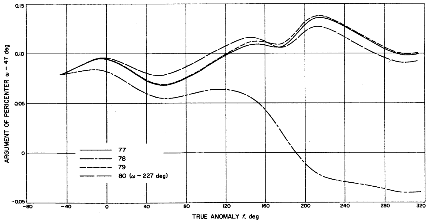
Fig. 5. Argument of pericenter
