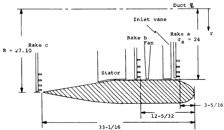
Longitudinal Section
