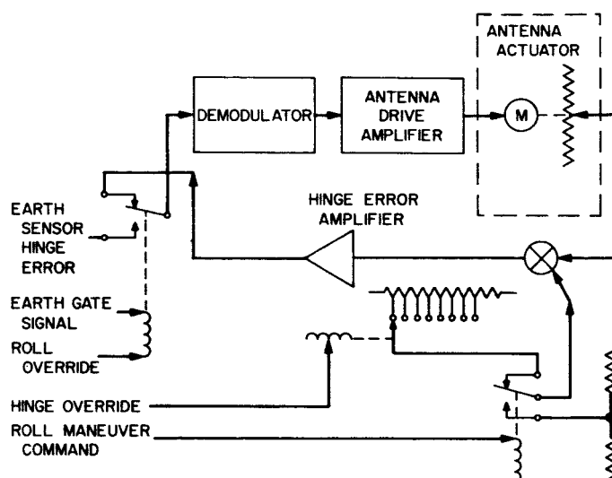
Fig. 7. Hinge servo loop
