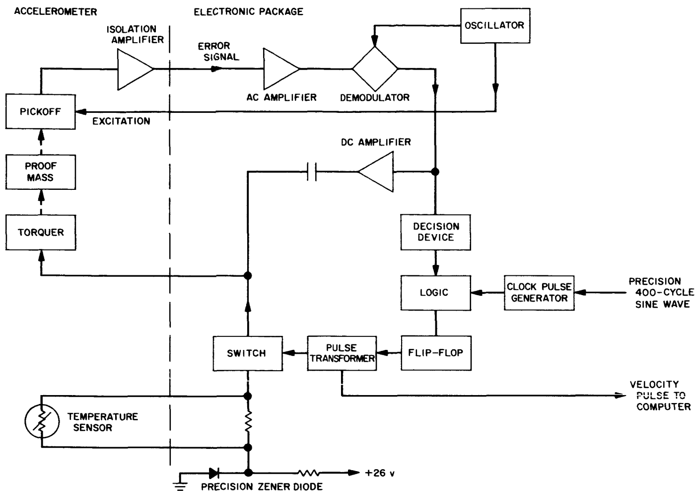
Fig. 61. Accelerometer subsystem
