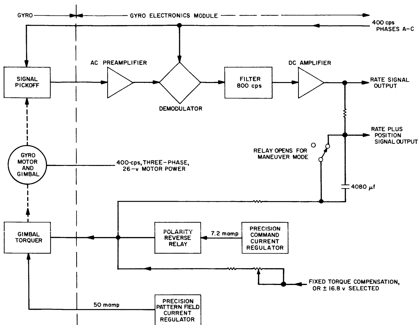
Fig. 9. Ranger gyro loops
