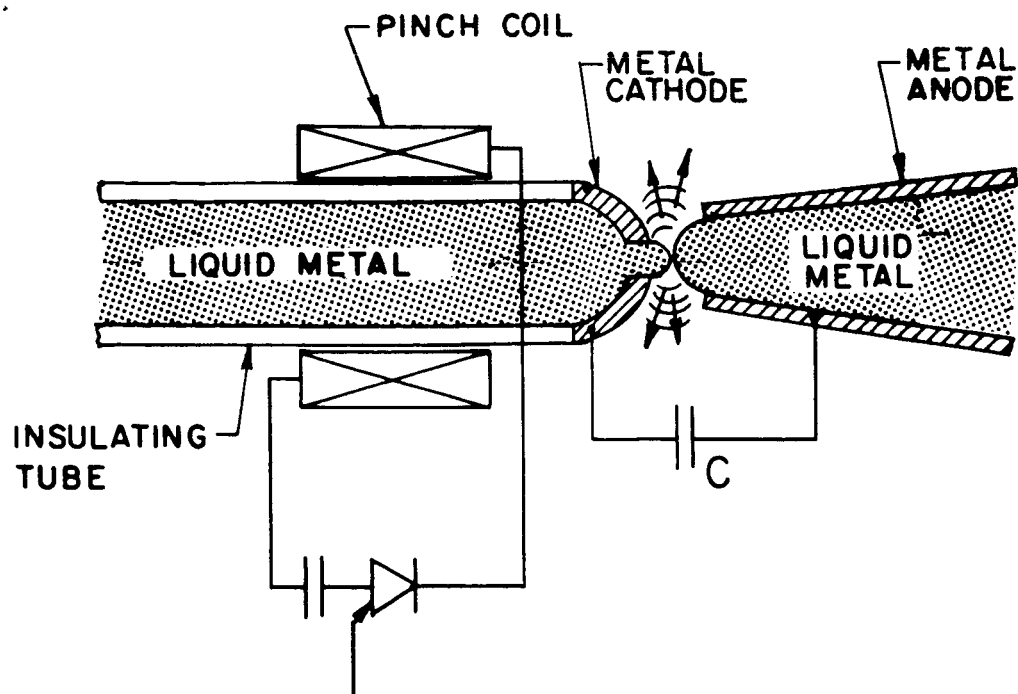
FIG. 35 : METAL PROPELLANT INJECTOR
