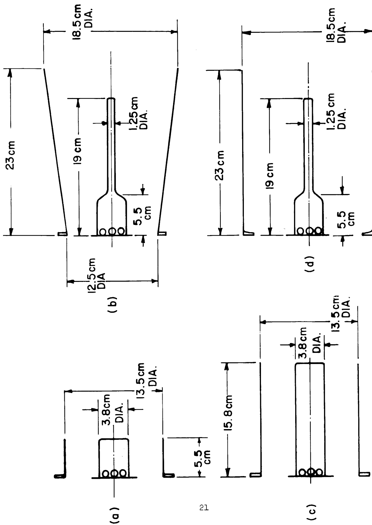
FIG. 11 : BARREL CONFIGURATIONS
