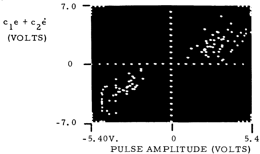
FIGURE 4 - c_1e + c_2\dot{e} Vs PULSE AMPLITUDE FOR OPTIMAL PARAMETER VALUES
