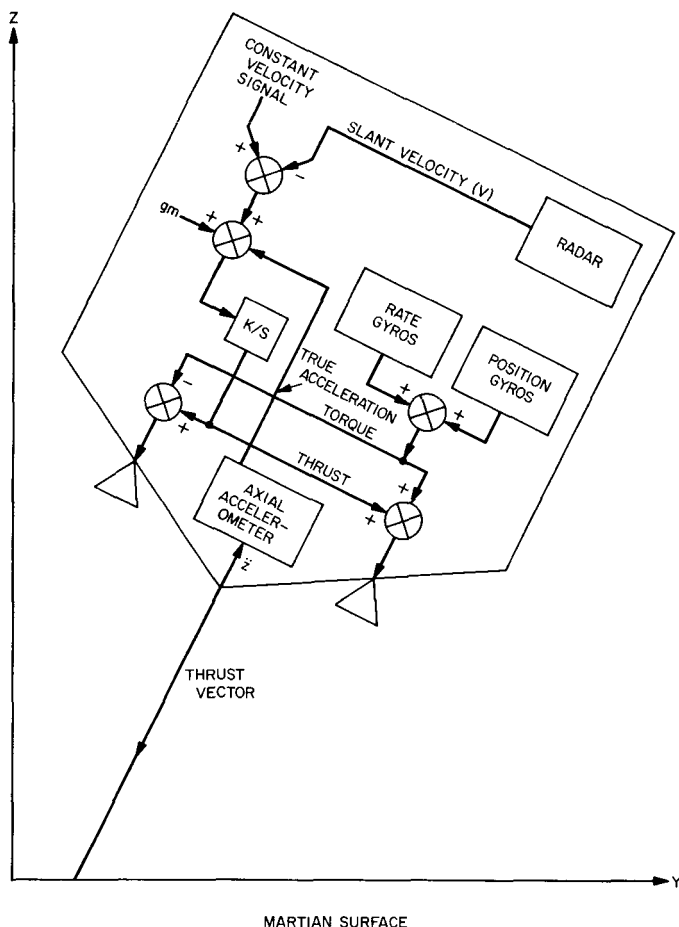
Fig. 7. Terminal mode
