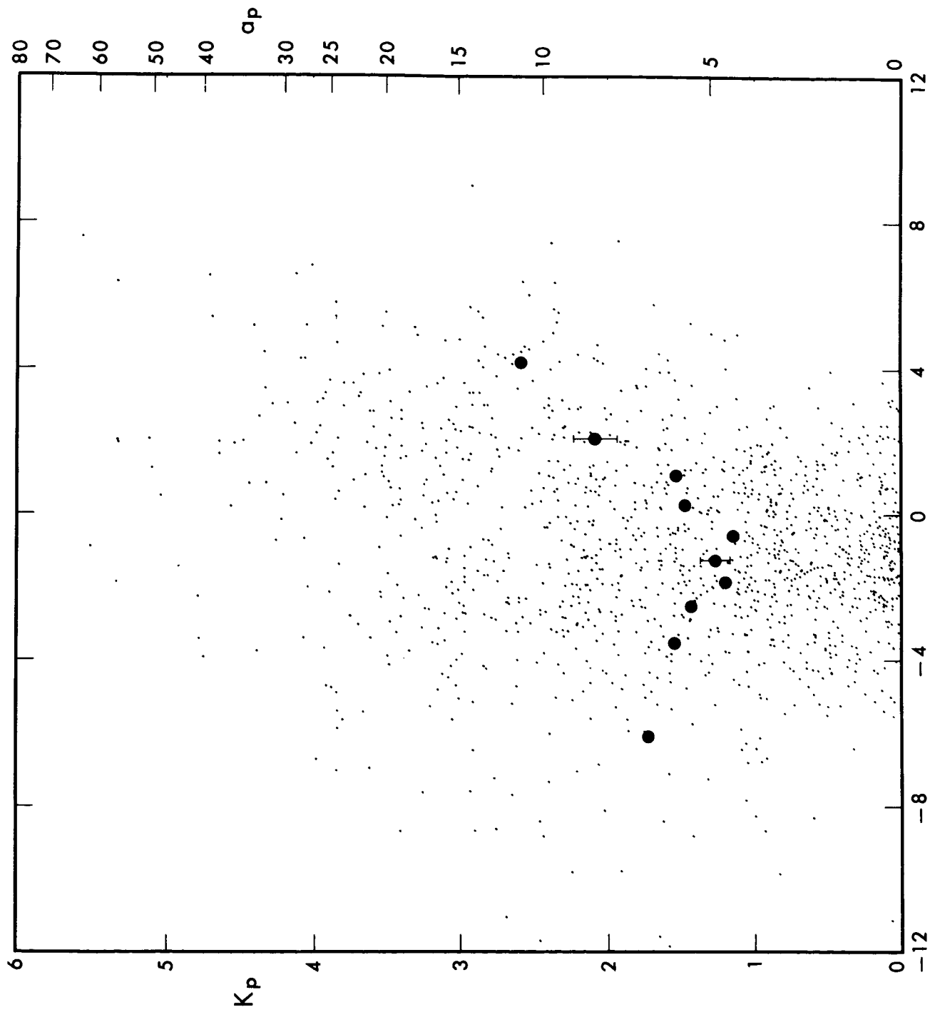
B_\phi , GAMMAS
