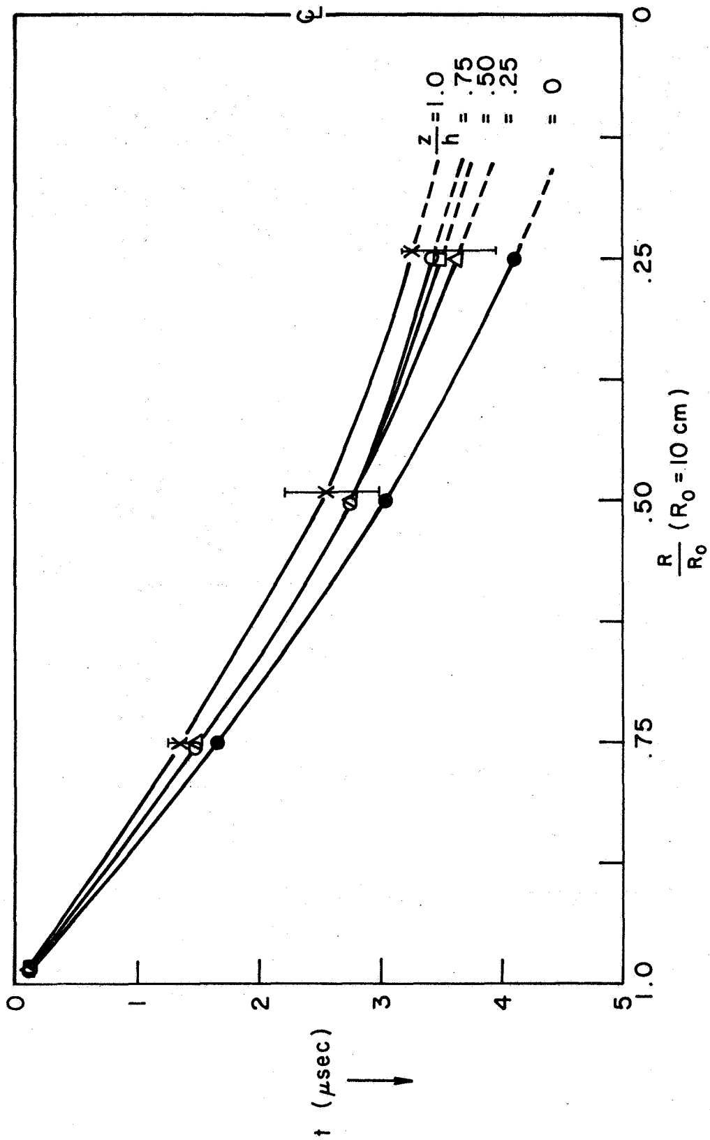
\dot{B}_\theta TRAJECTORIES
