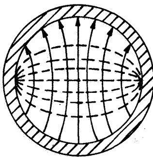
b. TE_{11} MODE
