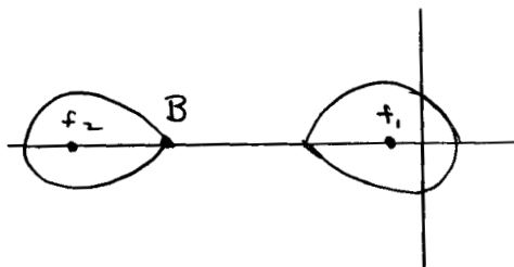
fig. 1a a_1 > 0, a_2 > 0
