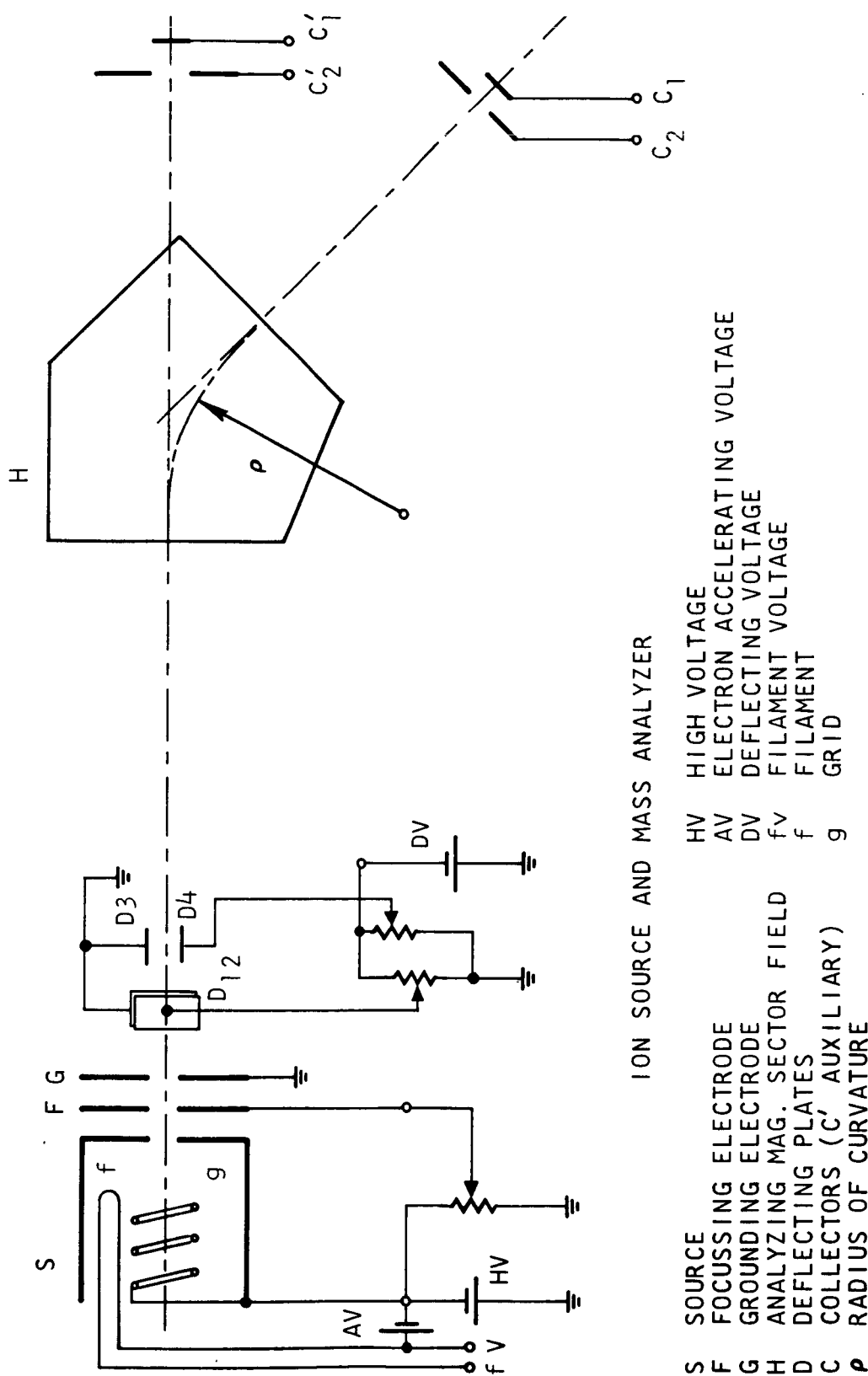
Fig. 10--Ion source apparatus
