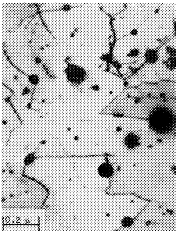
(d) Ni-33.7Cr-1ThO 2
