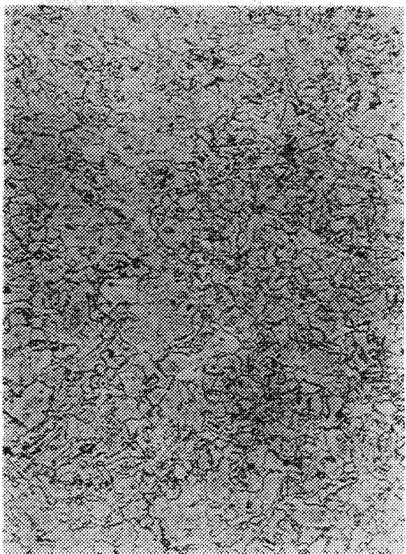
(d) Ni-33.7Cr-1ThO 2
