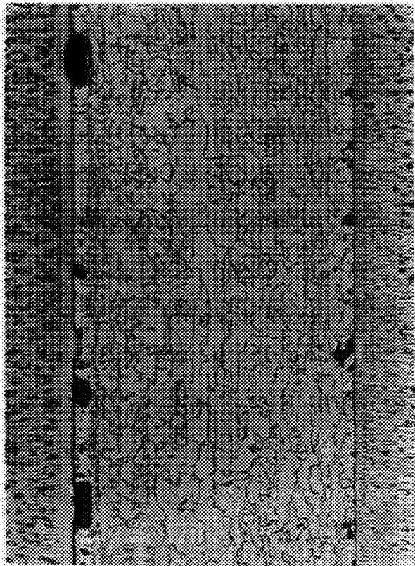
(d) Ni-33.7Cr-1ThO 2
