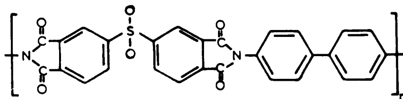
POLYMER A''
