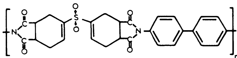
POLYMER A'
