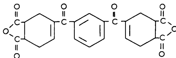
MONOMER E
