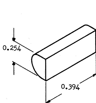
P - Pellet
