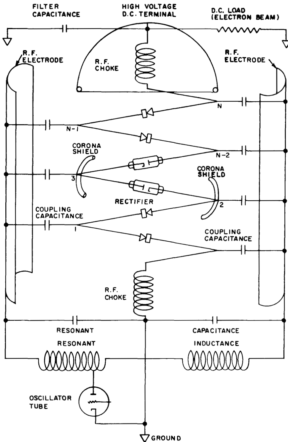
FIG. 3 : DYNAMITRON ACCELERATOR
