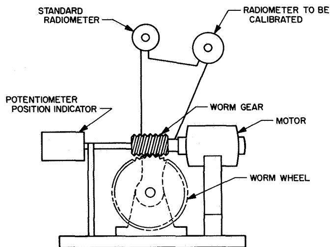
Fig. 8. Radiometer positioner
