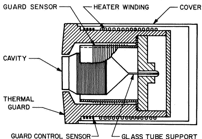
Fig. 1. Standard radiometer
