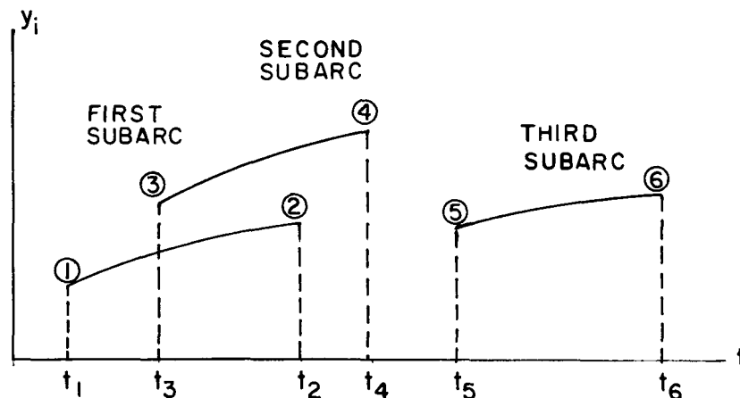
FIGURE 1.1 MULTIPLE SUBARCS
