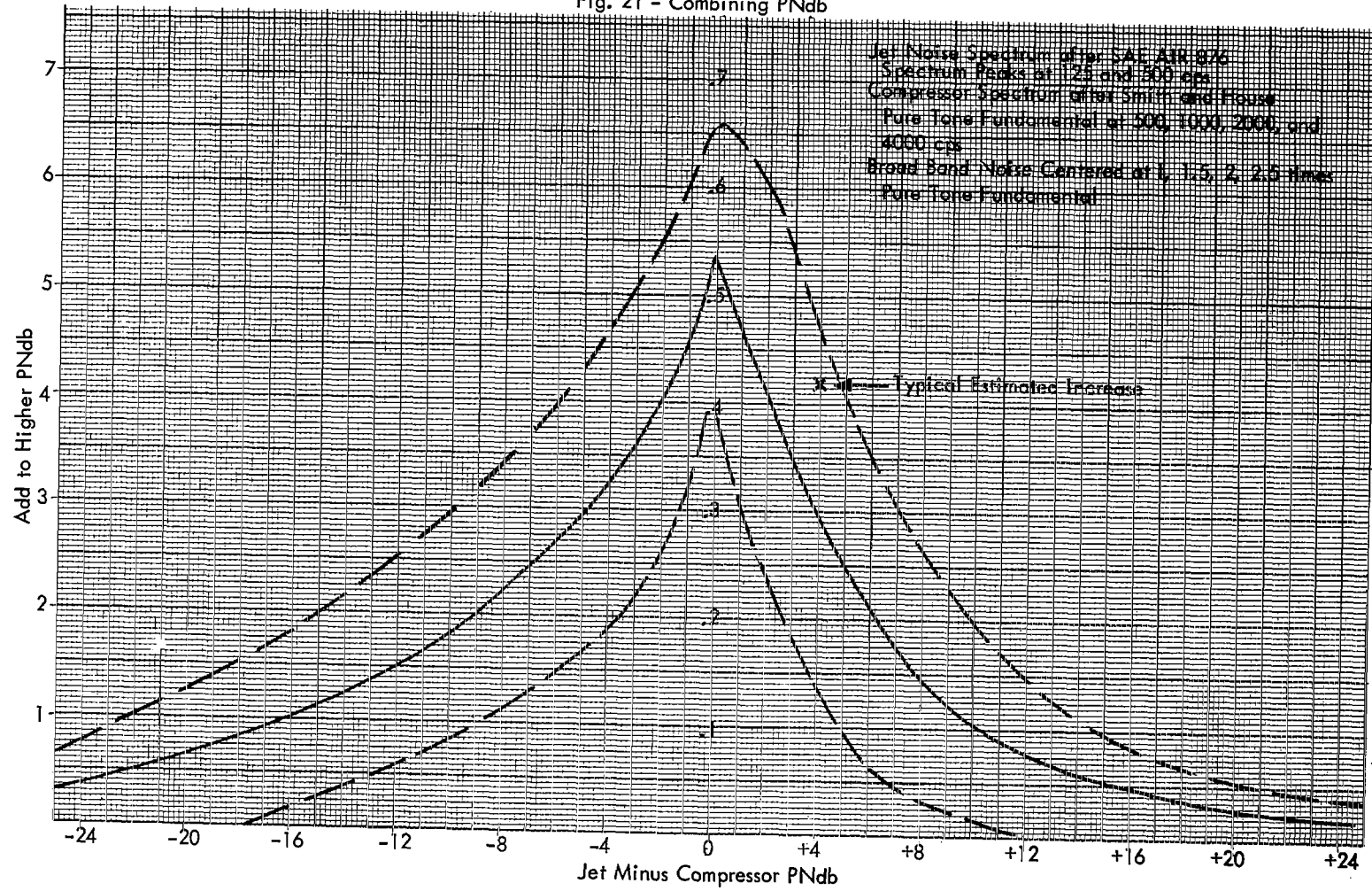
Fig. 21 - Combining PNdb
