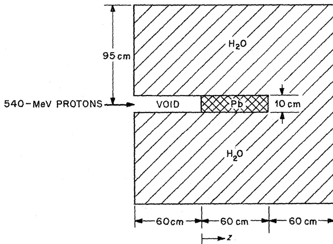
Fig. 1. ING Experiment.
