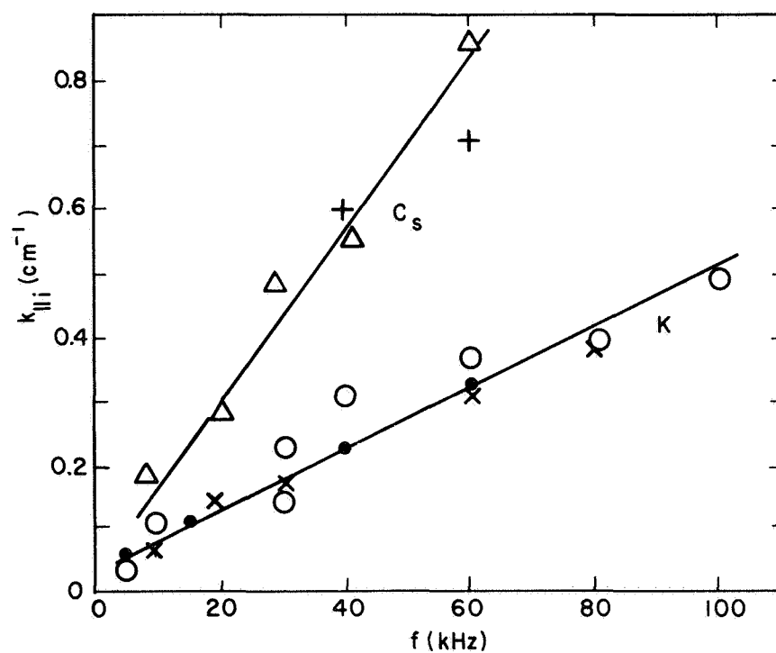
(b) ATTENUATION
