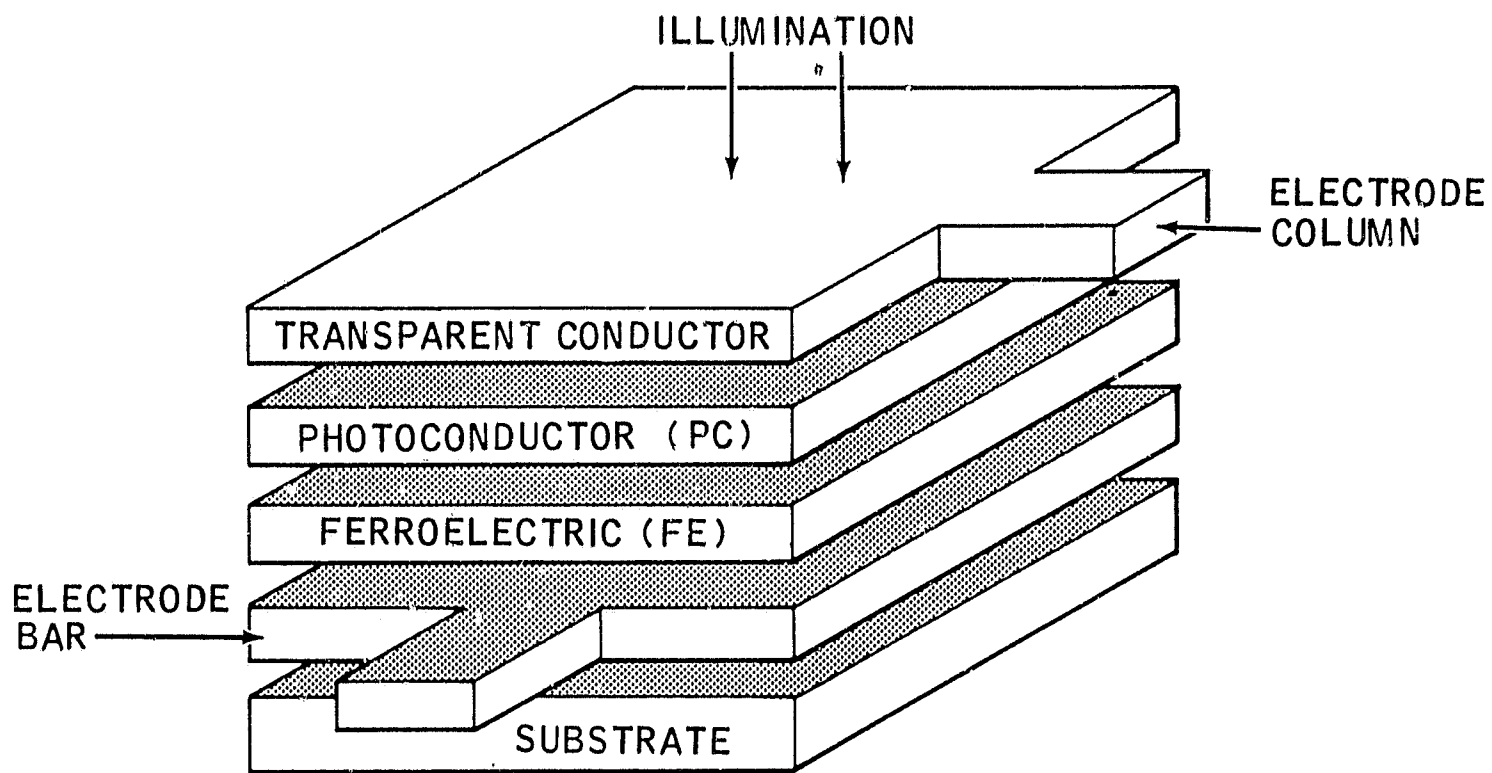
A. LAMINATE
