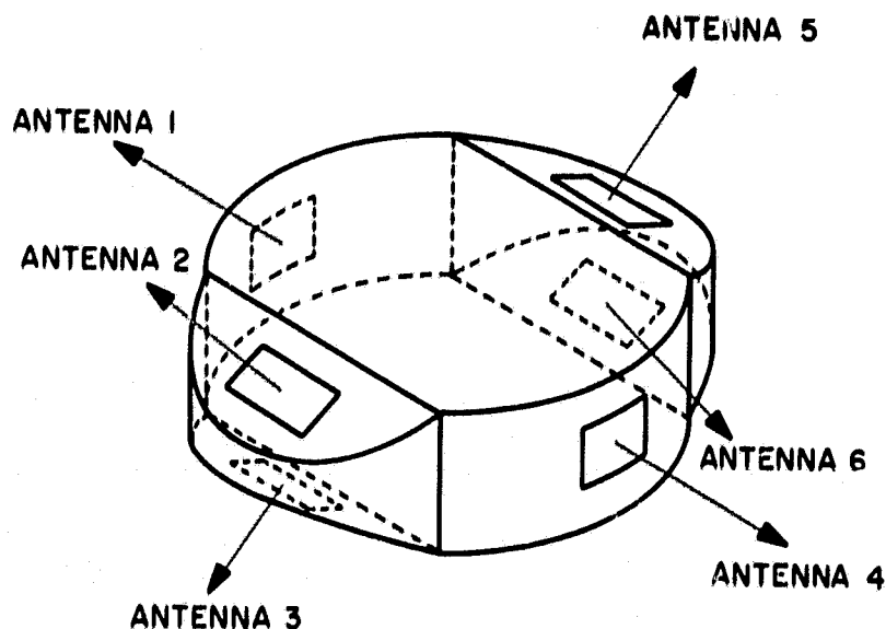
Fig. 1. JPL CSAD lander antenna configuration
