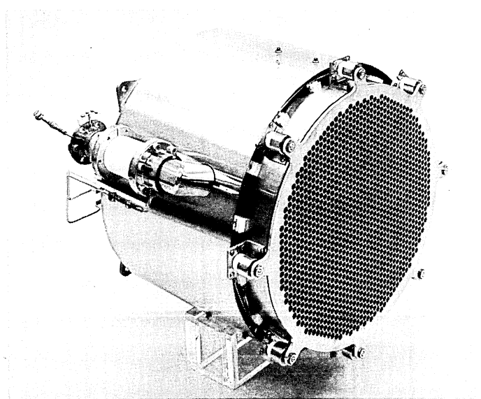
Fig. 1. A 20-cm-diam ion thruster
