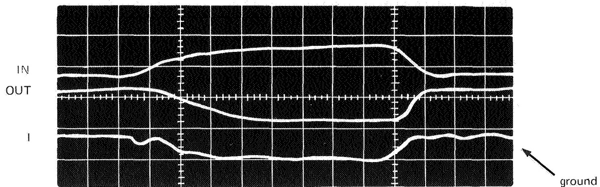
2N 4352 P-channel
