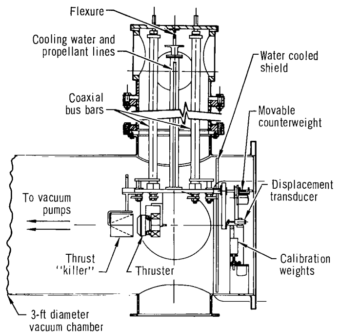
Fig. 3.1 Thrust stand
