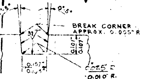
DETAIL "A" SCALE: 48" = 1'-0"
