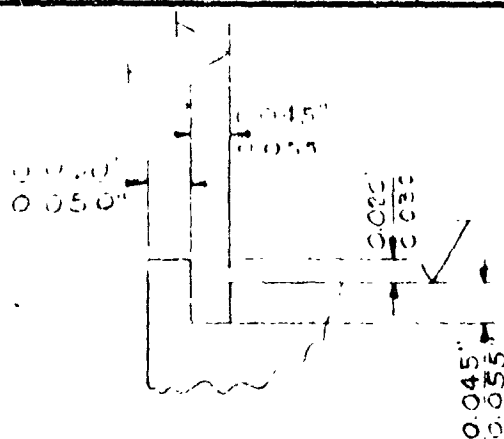
DETAIL "A" SCALE: 48"=1'-0"
