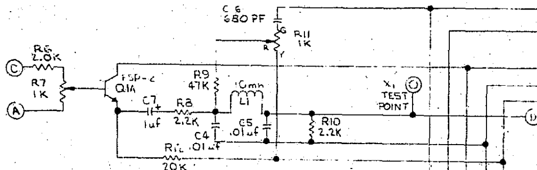
X-1 BRIDGE CKT
