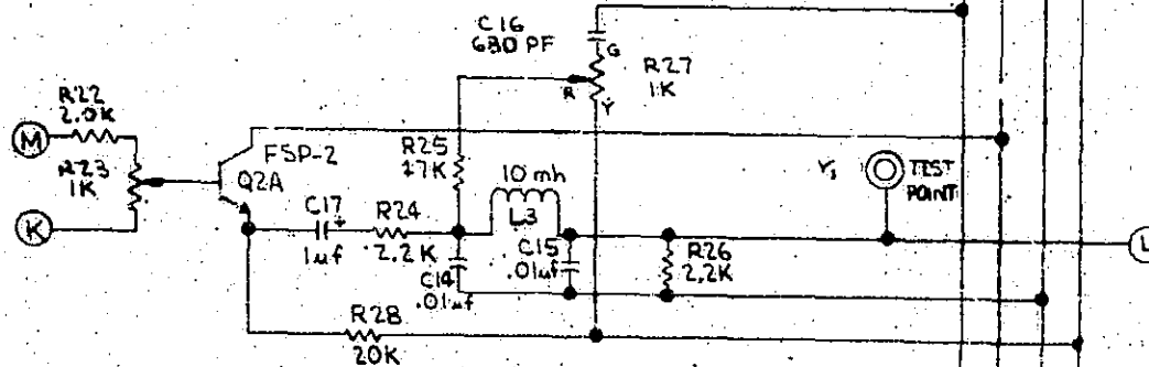
Y-1 BRIDGE CKT
