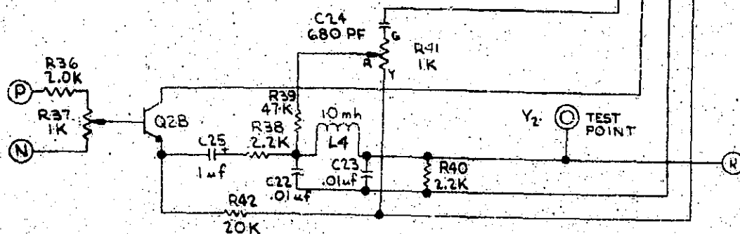
Y-2 BRIDGE CKT
