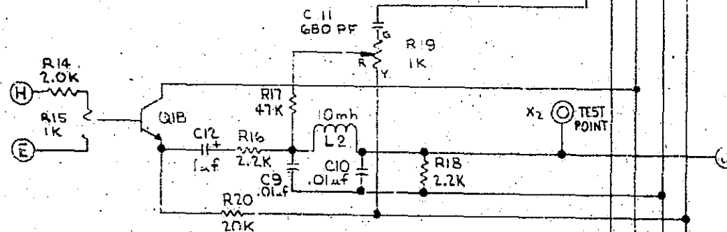
X-2 BRIDGE CKT
