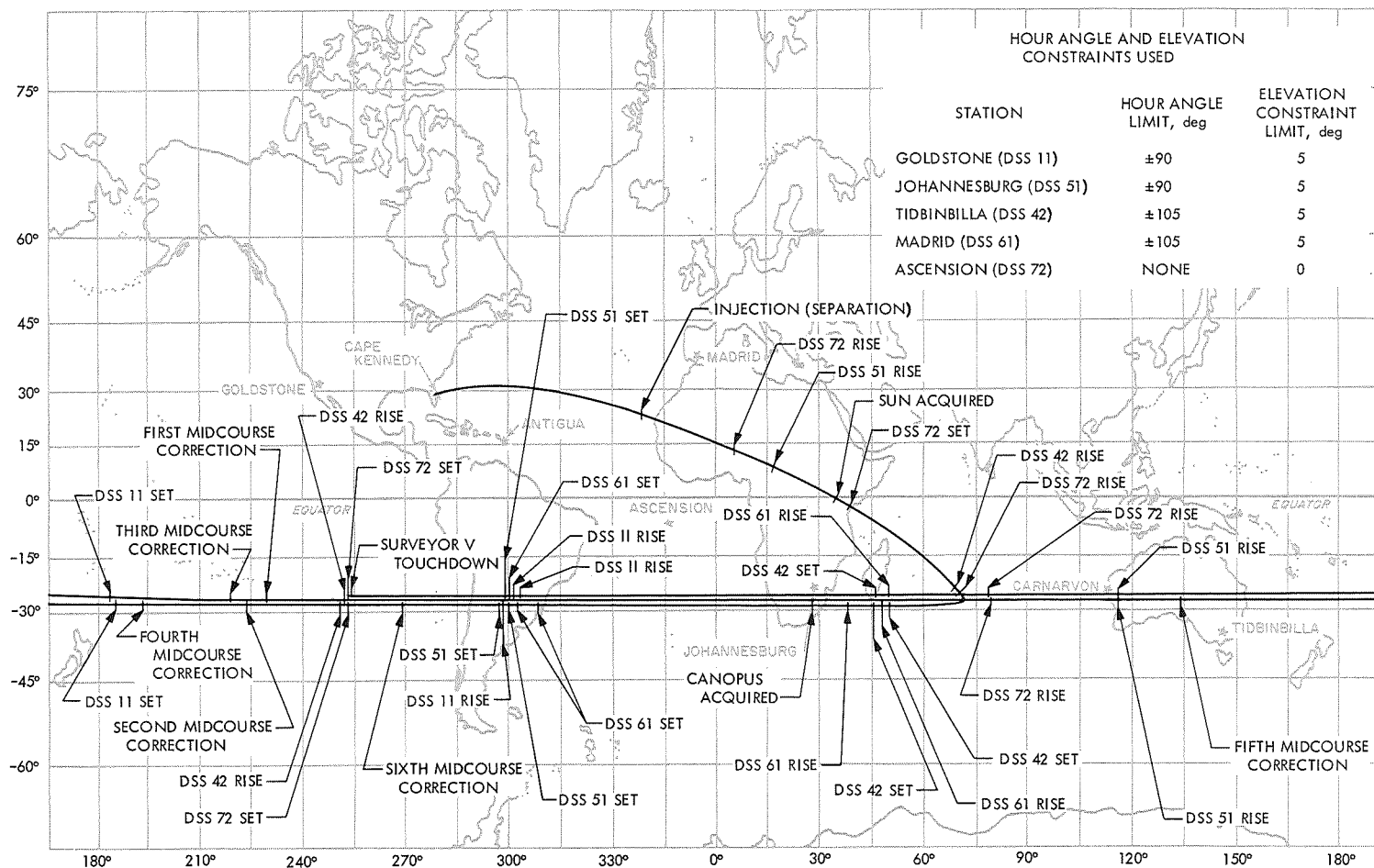
Fig. 26. Surveyor V actual earth track
