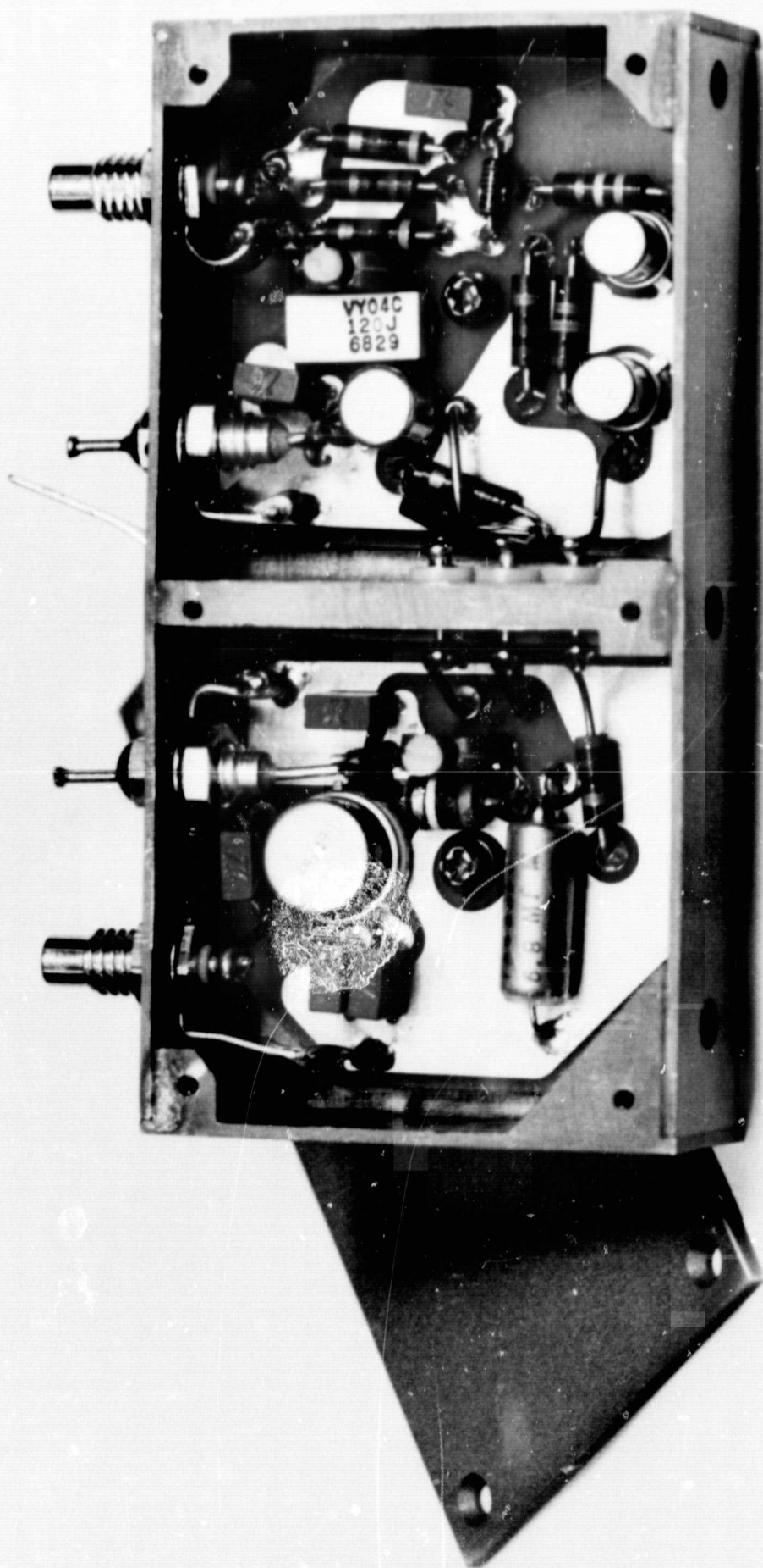
RF AMPLIFIER MODULE
