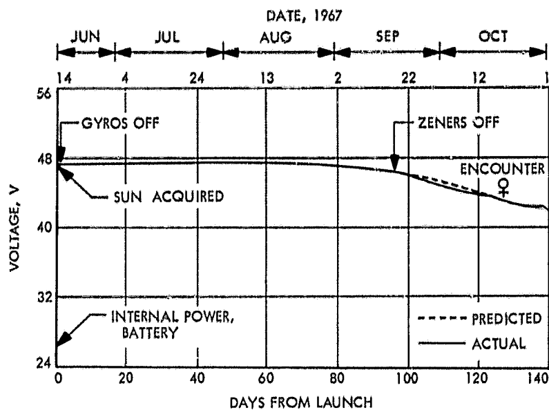
Fig. 33. PS&L voltage
