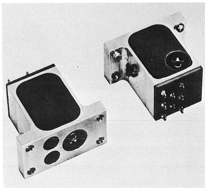
Fig. 18. Landing-sensor module
