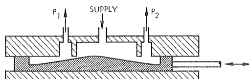
(d) LINEAR DISPLACEMENT WITH VARIABLE ORIFICES
