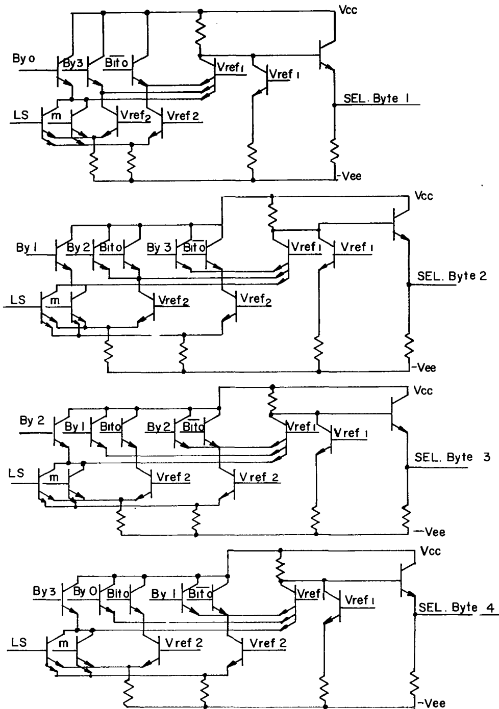
Fig. 4.2-7 BYTE SELECT
