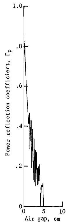
(d) Ka-band (12.7 cm × 12.7 cm reflector).
