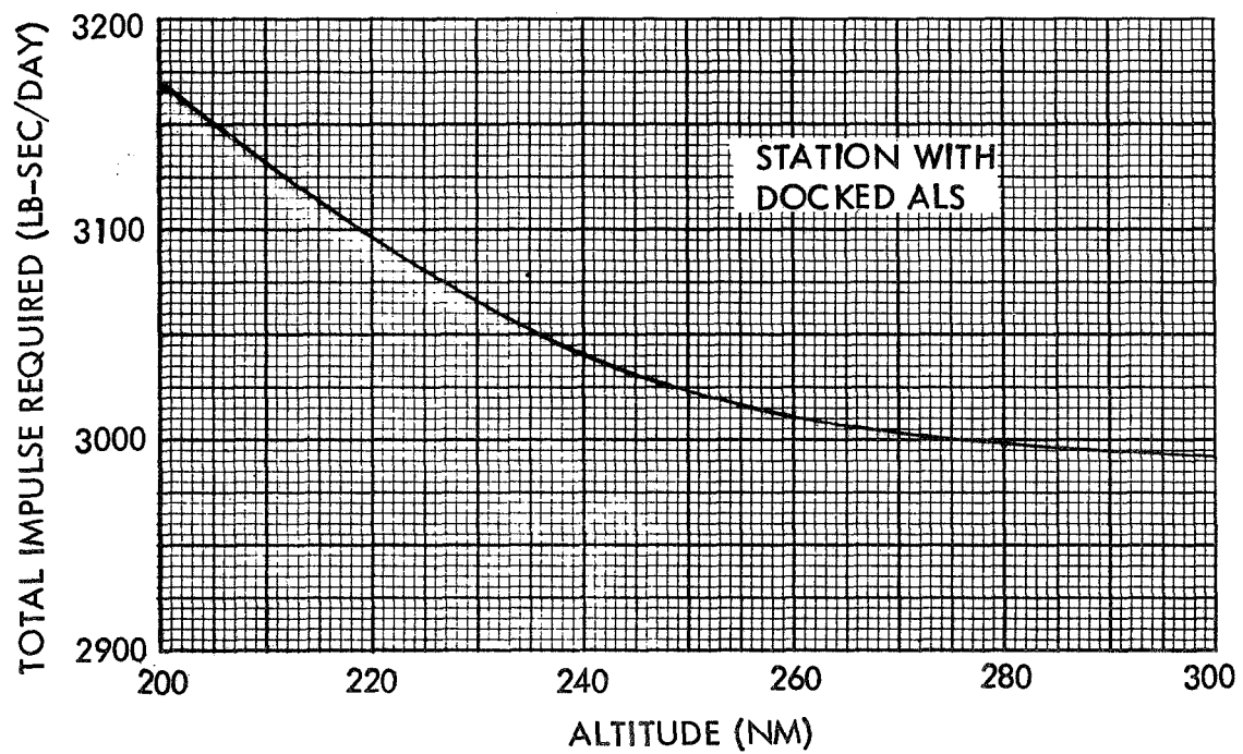
Figure 3-15. Gravity Gradient Impulse, With ALS
