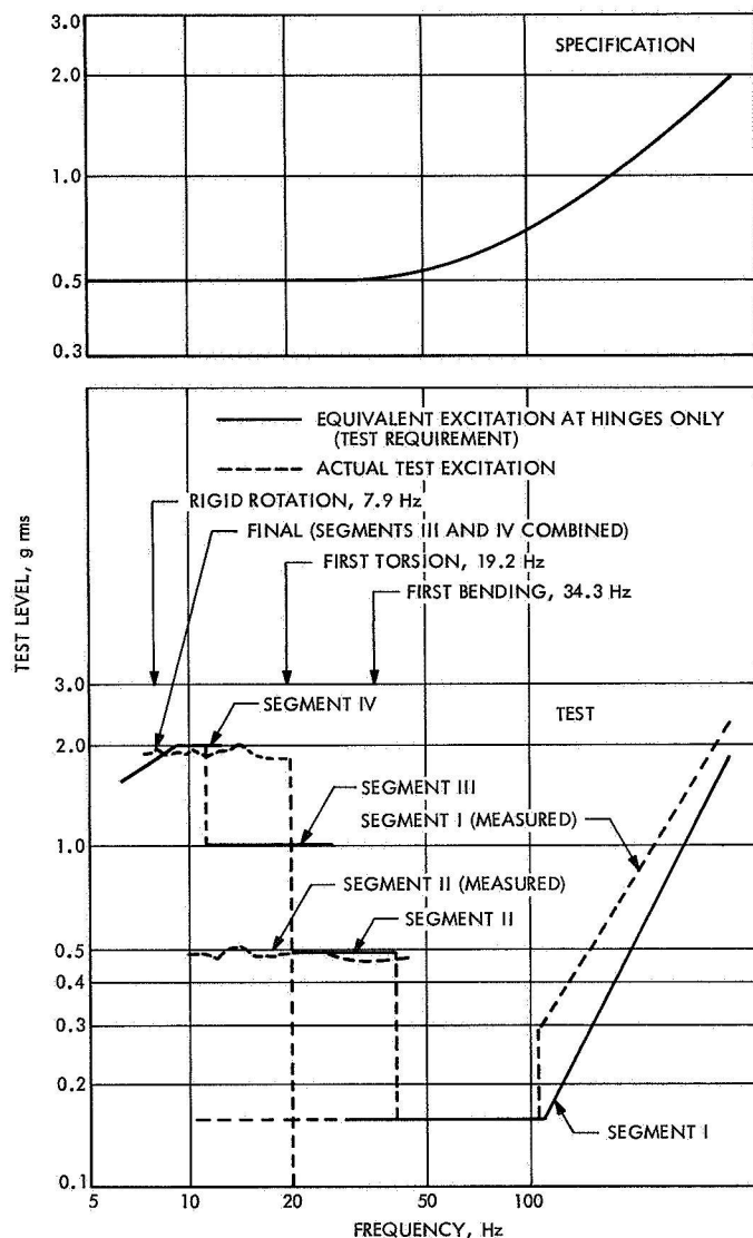
Fig. 20. Sinusoidal vibration test levels
