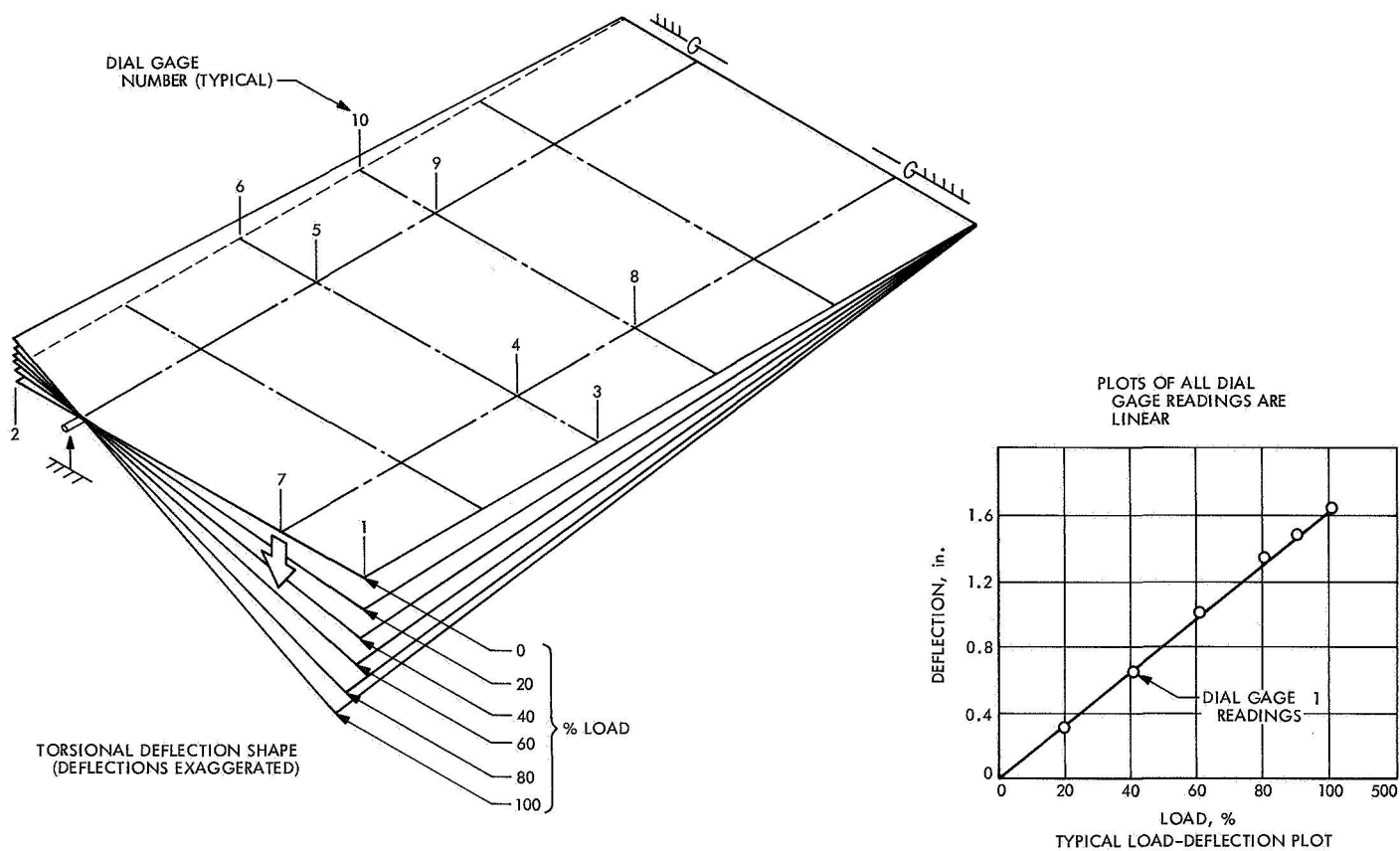
Fig. 22. Deflections – 50-lb load
