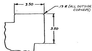
DETAIL A TYP 4 PLACES SCALE: 1/2
