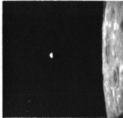
AS11-41-6038
