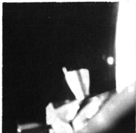
AS11-37-5439
