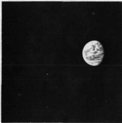
AS11-36-5330
