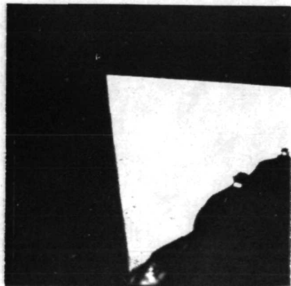
AS11-39-5788
