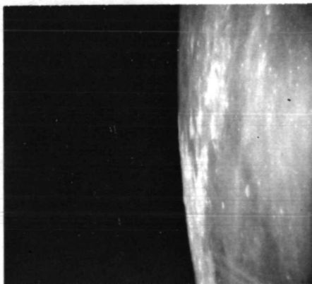
AS11-41-6071
