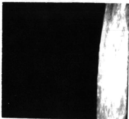
AS11-41-6001
