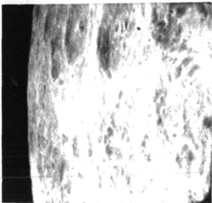
AS11-43-6515
