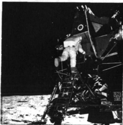
AS11-40-5866
