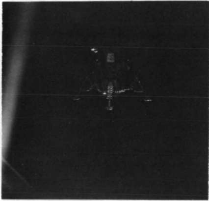
AS11-44-6590
