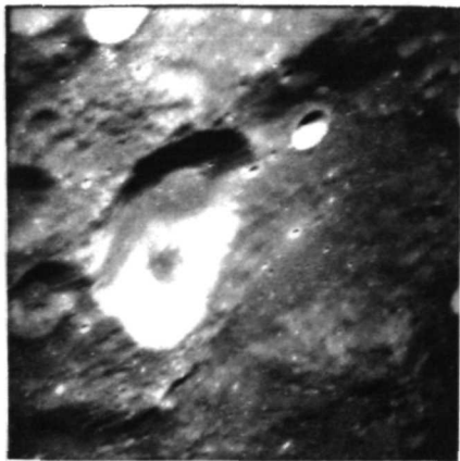
AS11-43-6403
