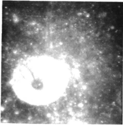
AS11-42-6286
