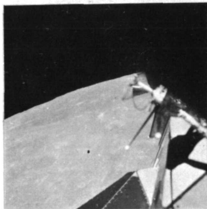
AS11-36-5418
