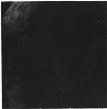
AS11-44-6690
