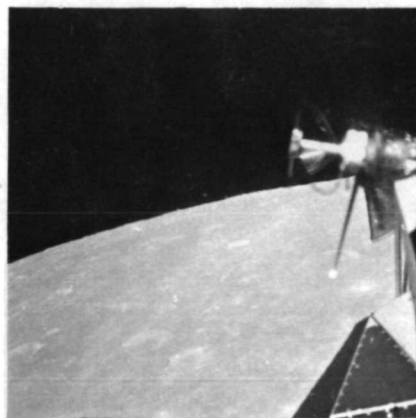
AS11-36-5414
