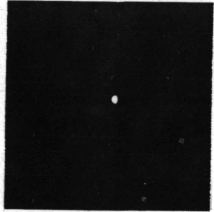
AS11-40-5845
