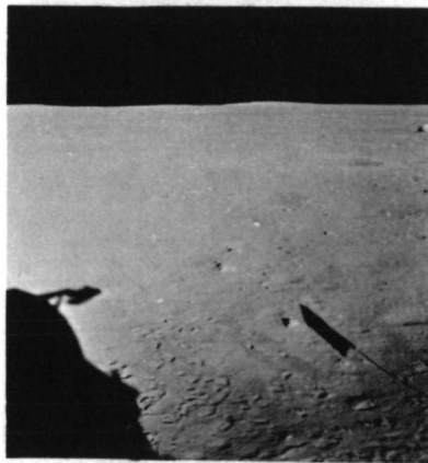
AS11-37-5465
