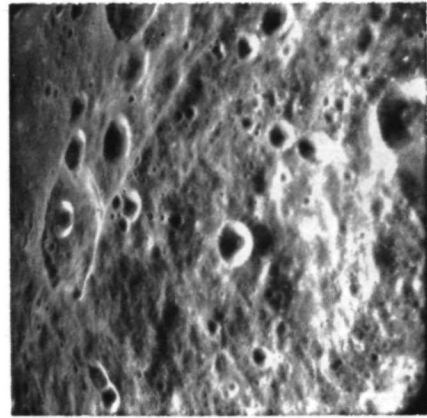
AS11-43-6506
