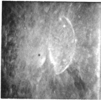
AS11-42-6336
