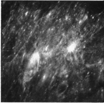
AS11-42-6294
