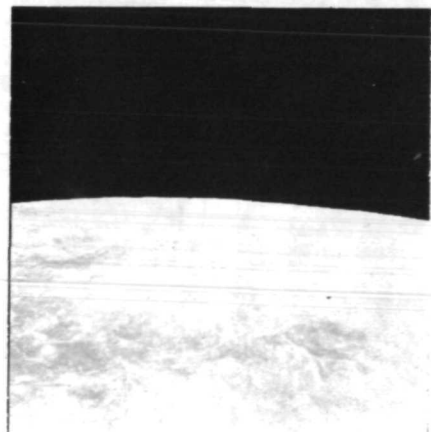
AS11-44-6545
