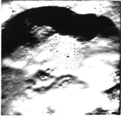
AS11-43-6391
