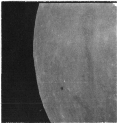
AS11-44-6658
