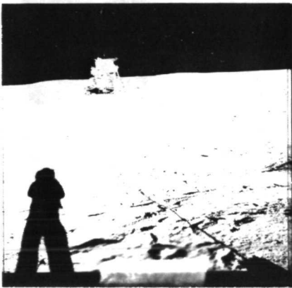
AS11-40-5961
