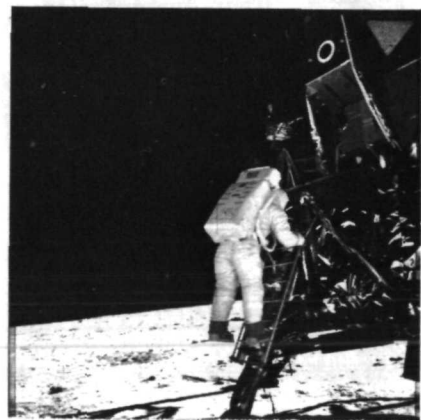
AS11-40-5867
