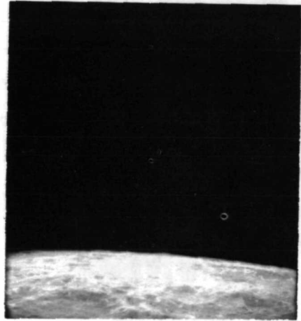
AS11-41-5984
