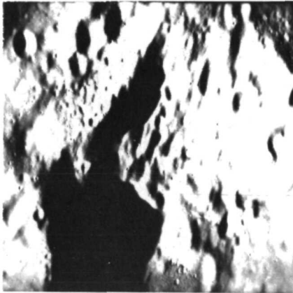
AS11-43-6381
