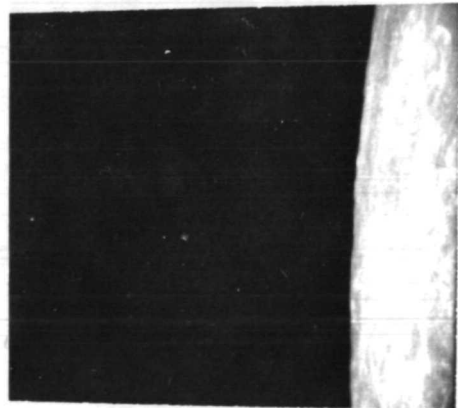
AS11-41-6000
