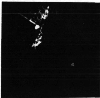
AS11-42-6272
