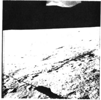
AS11-40-5960
