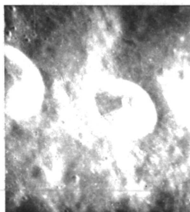
AS11-38-5579
