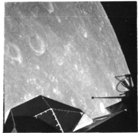
AS11-36-5430
