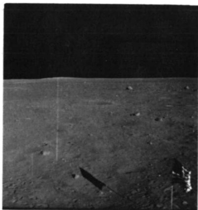
AS11-37-5511
