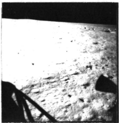
AS11-39-5781
