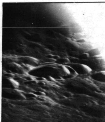
AS11-38-5559
