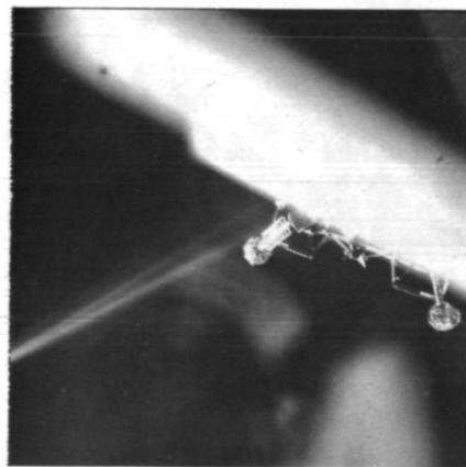
AS11-44-6569
