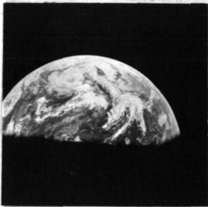
AS11-36-5321
