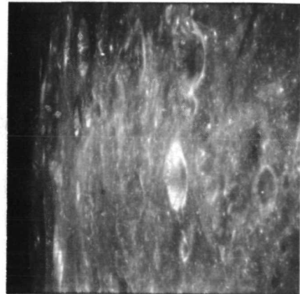
AS11-43-6352
