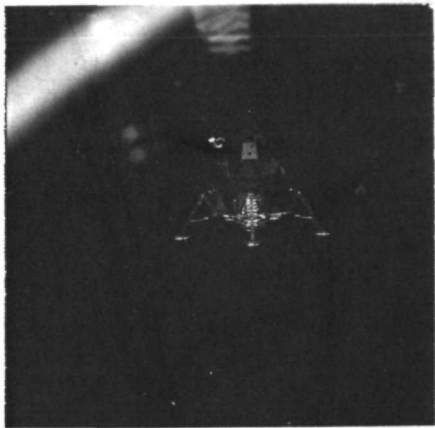
AS11-44-6594
