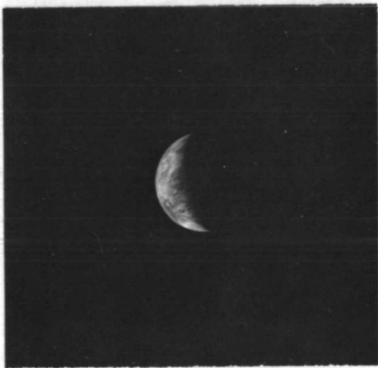
AS11-44-6676
