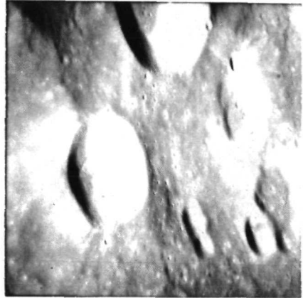
AS11-43-6400
