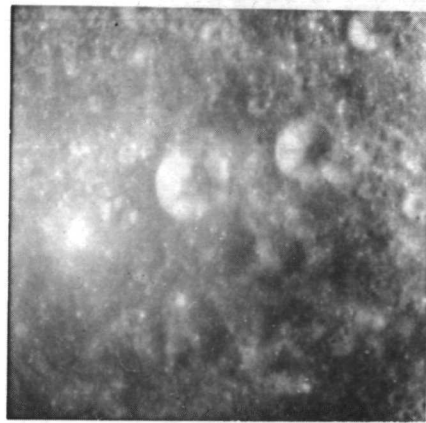
AS11-42-6257
