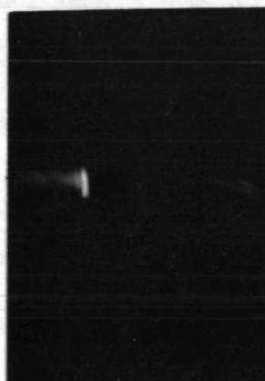
AS11-37-5438
