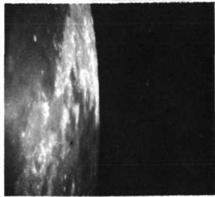
AS11-41-6074
