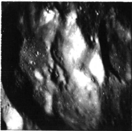
AS11-43-6393
