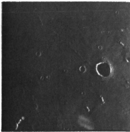
AS11-42-6238
