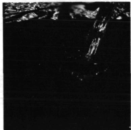
AS11-40-5896
