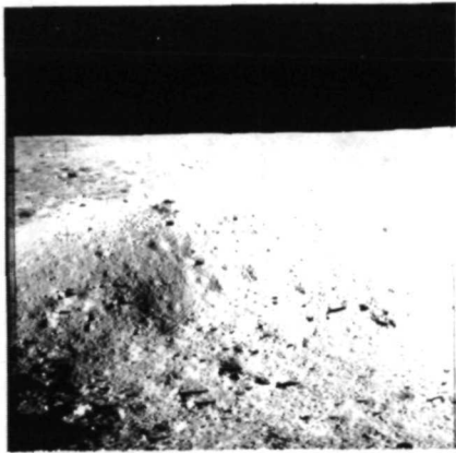
AS11-40-5891
