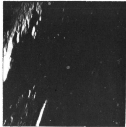
AS11-43-6368
