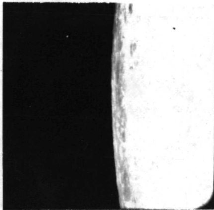
AS11-43-6529
