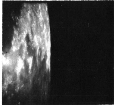
AS11-41-6076
