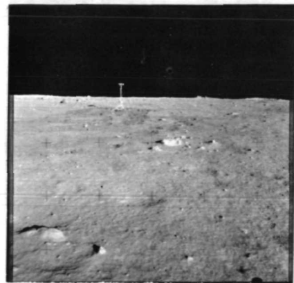
AS11-40-5908
