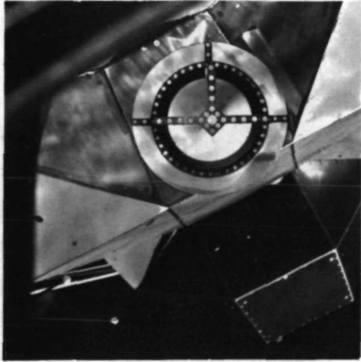
AS11-36-5365
