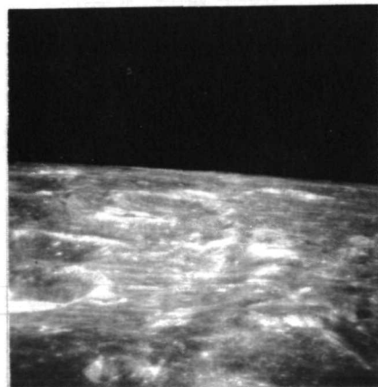
AS11-43-6360
