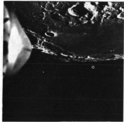
AS11-42-6235
