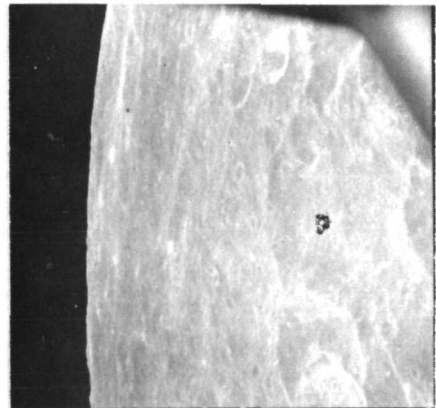
AS11-44-6621
