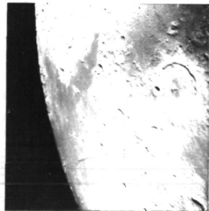
AS11-42-6231
