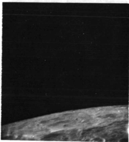
AS11-41-5975
