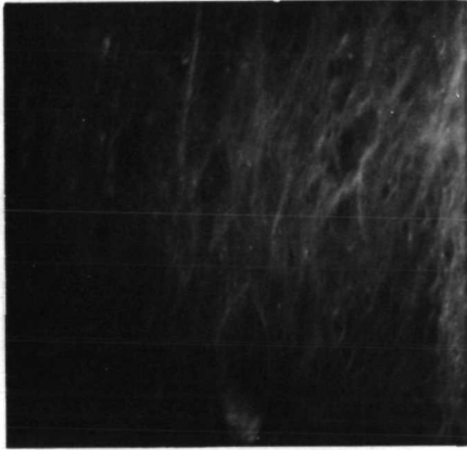
AS11-42-6330
