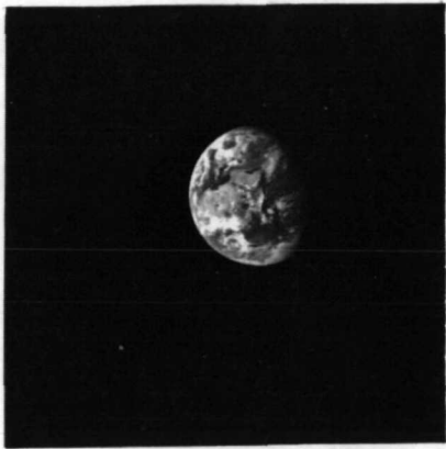
AS11-36-5353
