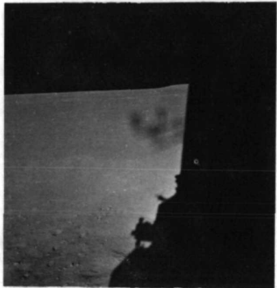
AS11-37-5496
