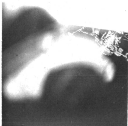
AS11-44-6572
