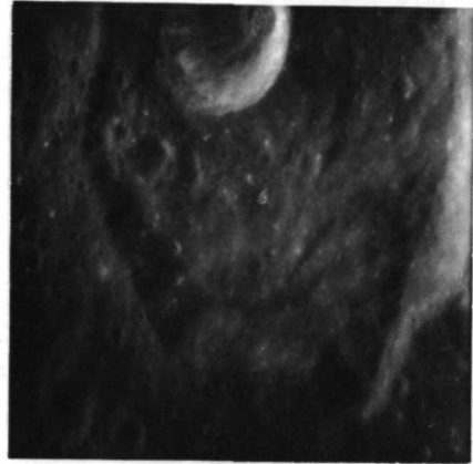
AS11-42-6329
