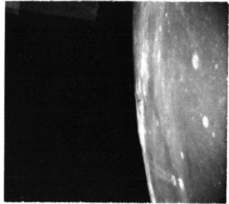
AS11-41-6068
