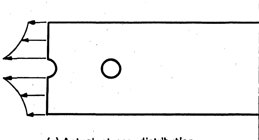
(a) Actual stress distribution
