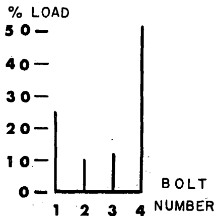
(d) Specimen 4
